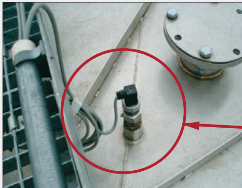
Место установки уровнемера ТИТАН-136У
